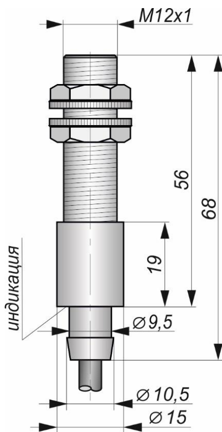
Габаритный чертеж
